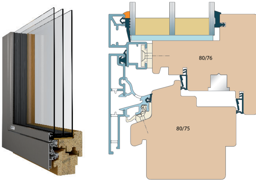
Darstellung: Bautiefe 95 mm Eiche / 3fach Isolierverglasung
